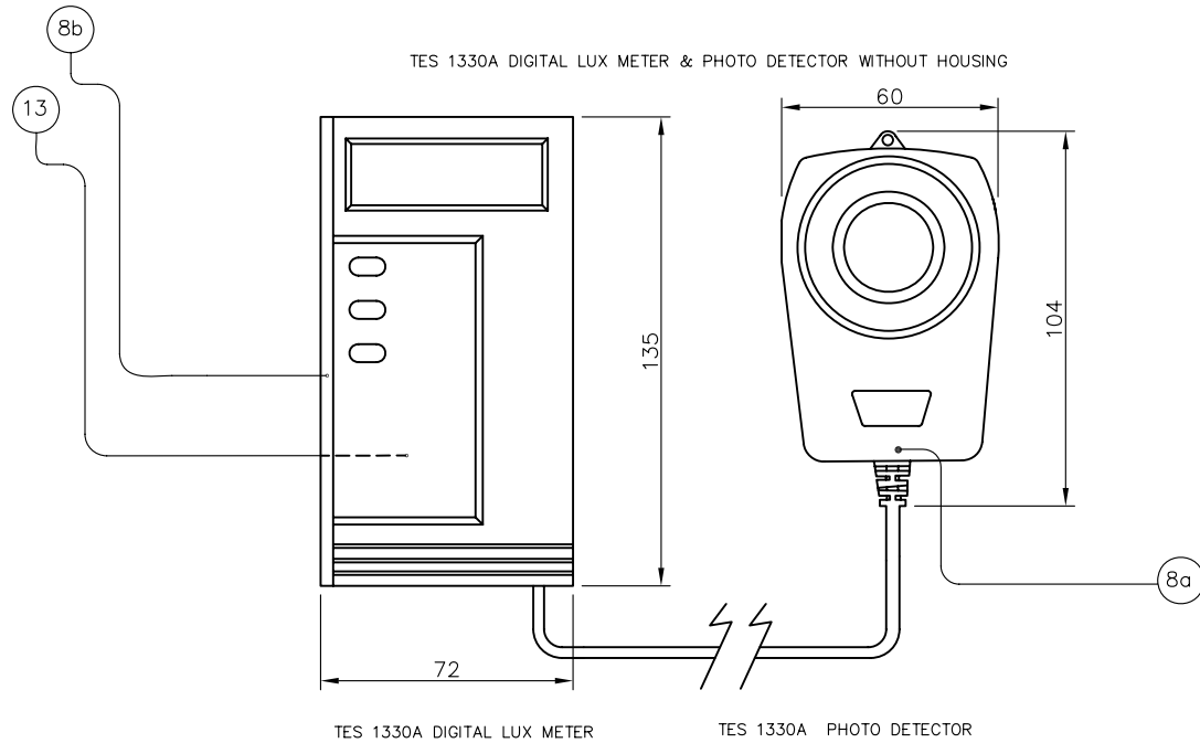
TES 1330A DIGITAL LUX METER
